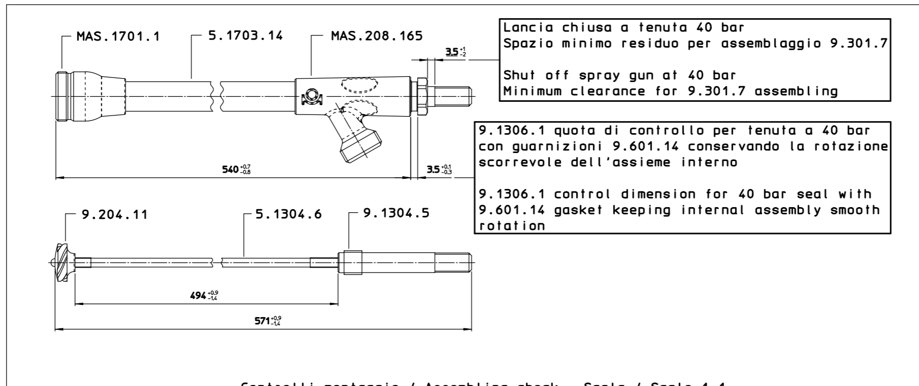
Controlli montaggio / Assembling check - Scala / Scale 1:1
